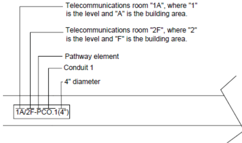
Pathway Label (conduit)
