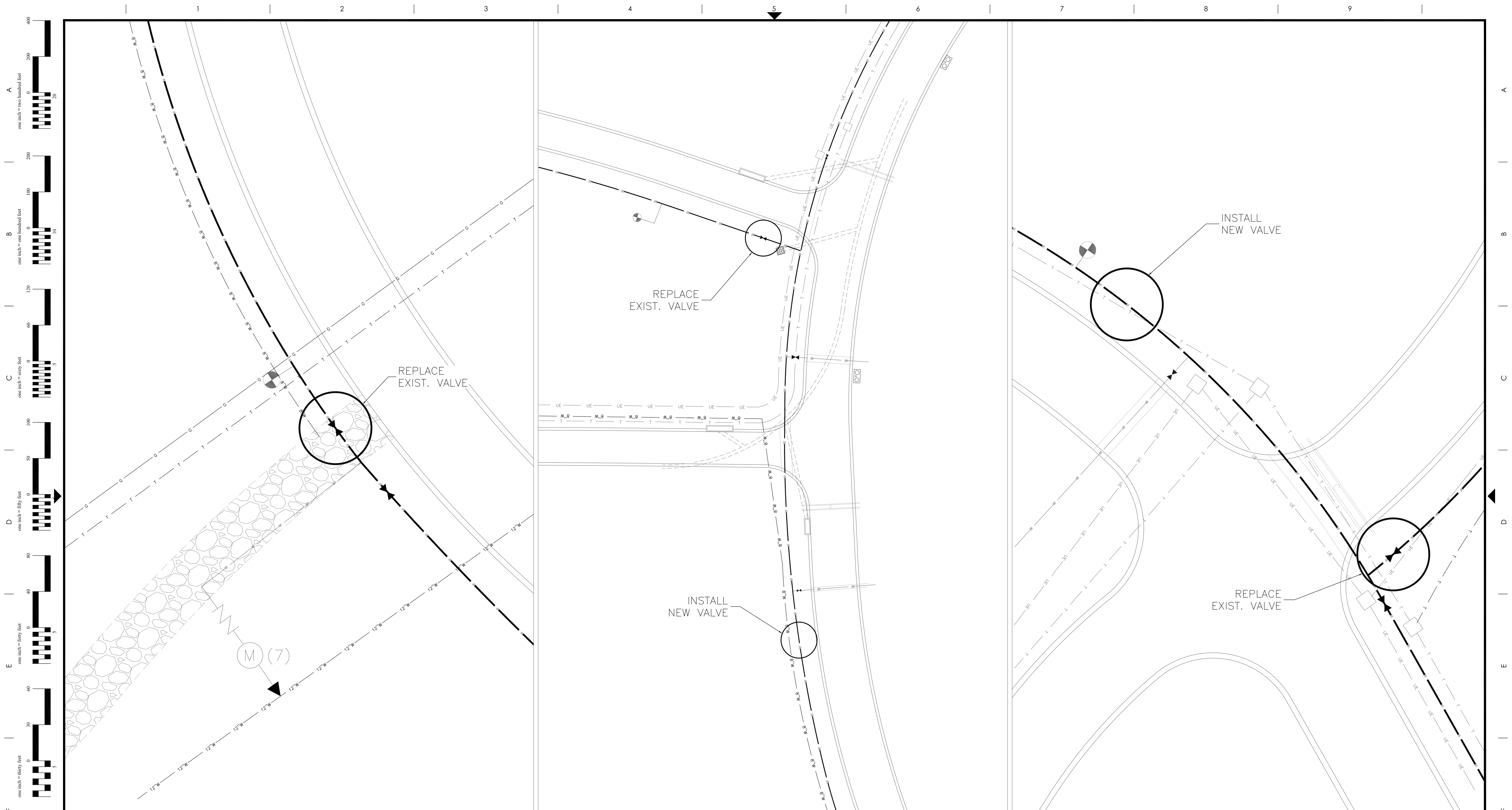
1 AREA 1 SITE PLAN L-102 SCALE: 1" = 10'-0"
